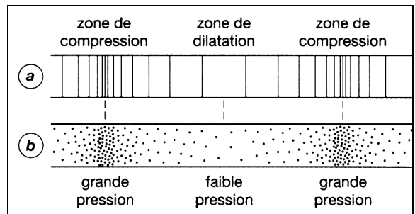
ondes sonores
