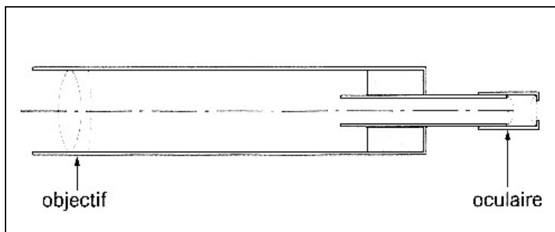
document n°2 : structure de la lunette astronomique
